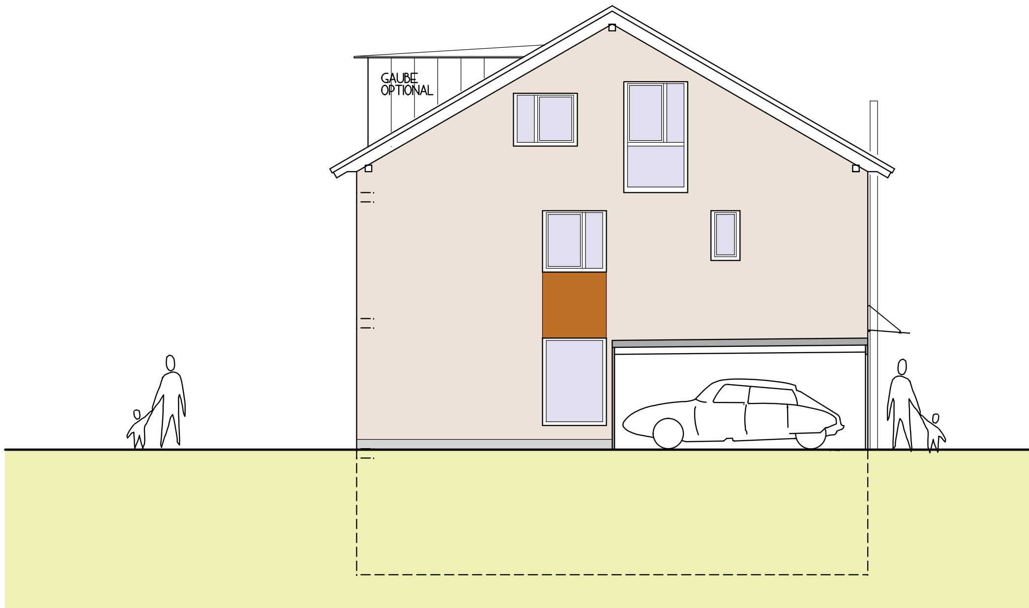
ANSICHT GIEBEL HAUS 2
